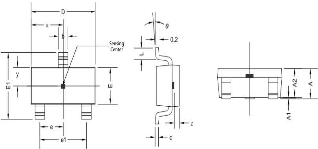
SOT23（Thin Outline）封装尺寸
