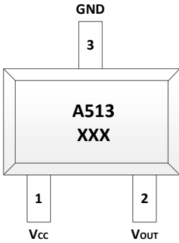
SOT23 (Thin)/SOT23-3L
